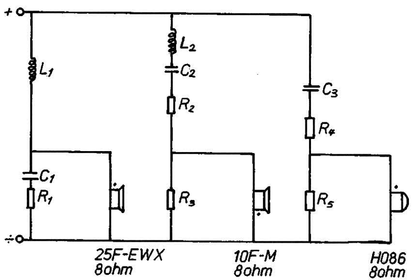
KOBLINGSSKJEMA. CIRCUIT DIAGRAM
